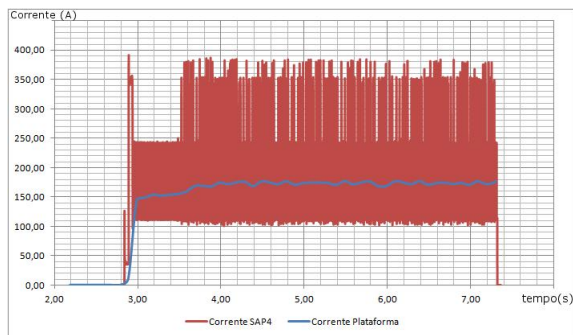
Figura 3: Gráfico de Corrente x Tempo
