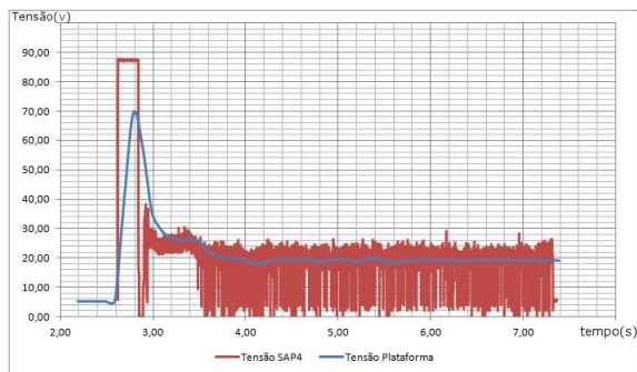
Figura 2: Gráfico de Tensão x Tempo
