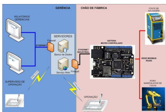
Figura 1. Modelo da Plataforma Proposta
